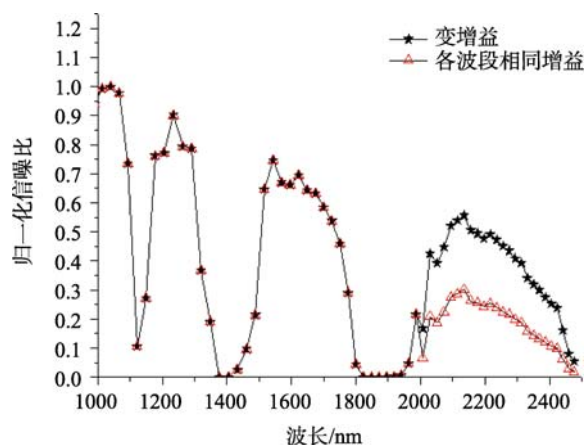
图6 探测器变增益设计对改善波段信噪比一致性的贡献
