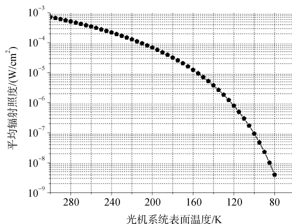
图4 不同光机系统表面温度对应的仪器背景辐射
